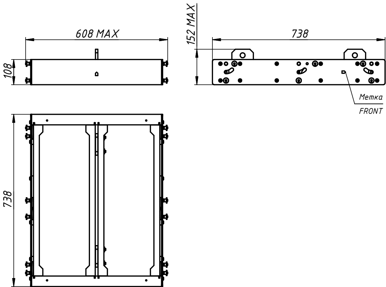
Габаритный чертеж
