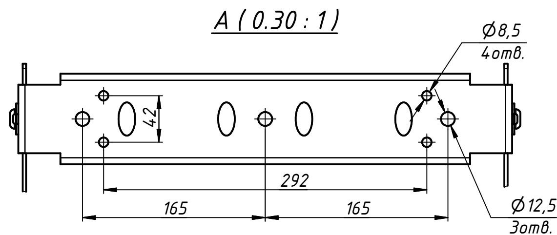
Точки крепления
