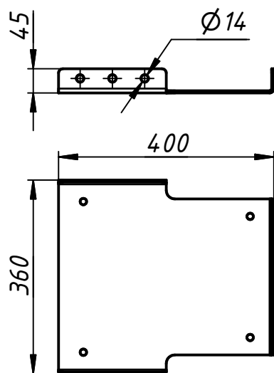
Отв. для подвеса
